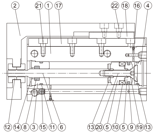
ø16, ø20
