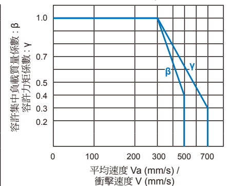
圖 4: 容許集中承載質量係數: \beta 容許力矩係數: \gamma
