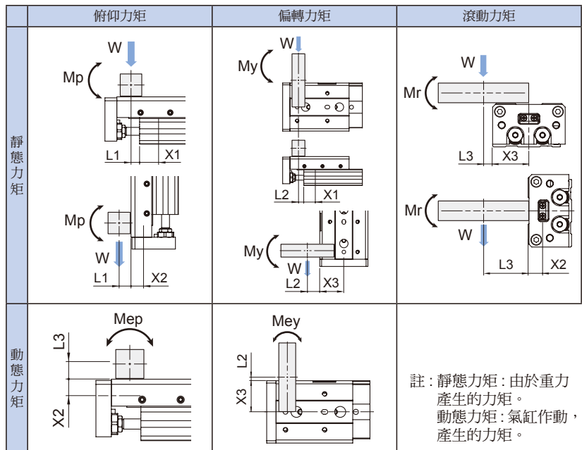
圖 2: 外伸量 : Ln (mm)，力矩中心位置距離修正值 : An (mm)
