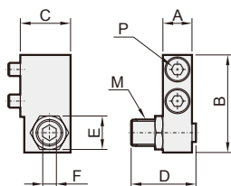
平台固定部
